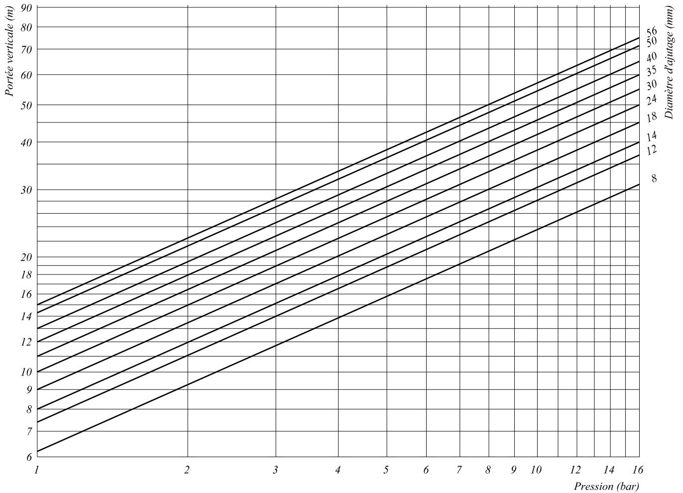
Portée verticale des lances d'incendie, en fonction de la pression et du diamètre d'ajutage
