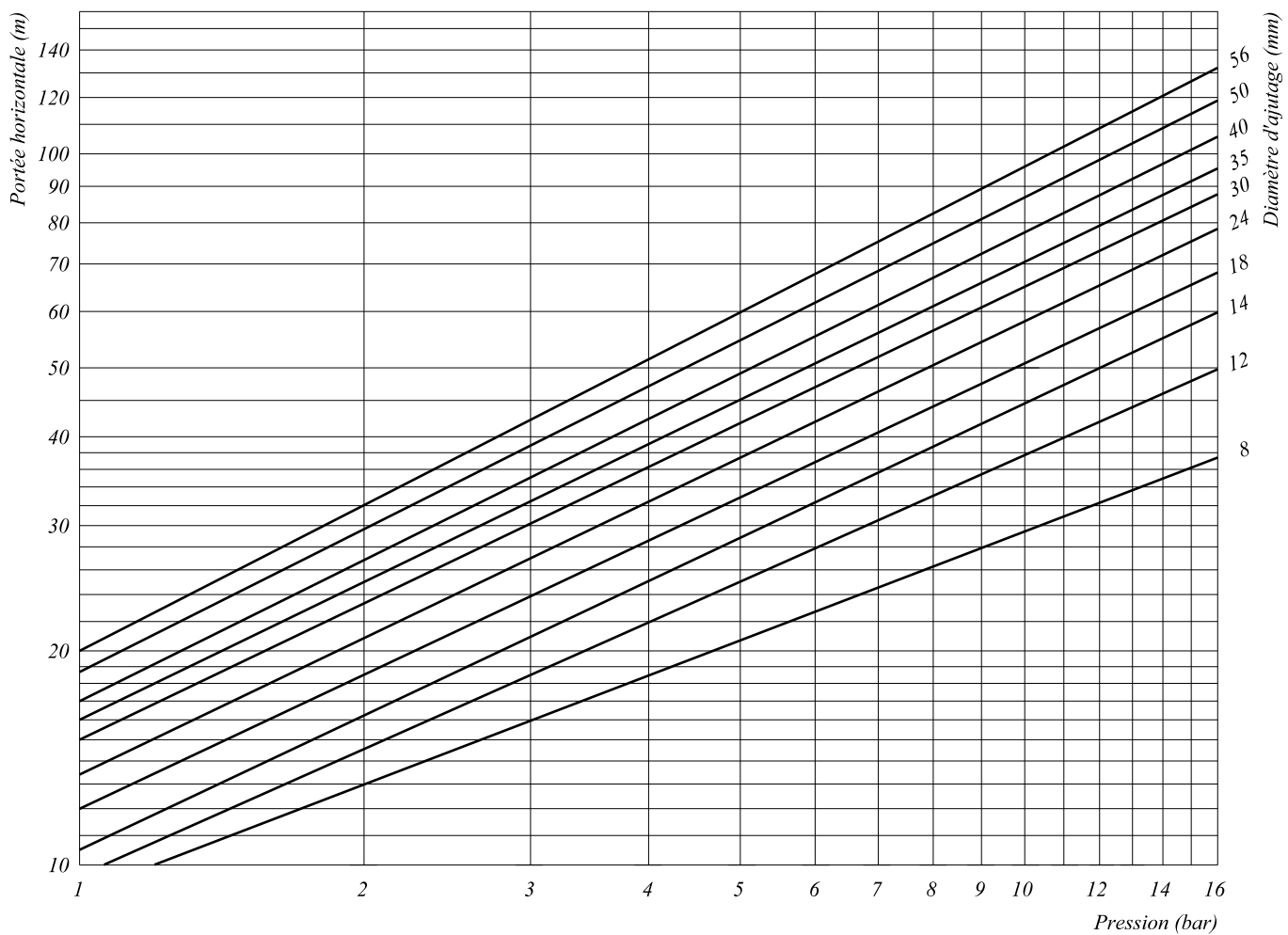
Portée horizontale des lances d'incendie, en fonction de la pression et du diamètre d'ajutage
